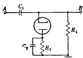
FIG. 4-9.—Diode d-c restorer.
